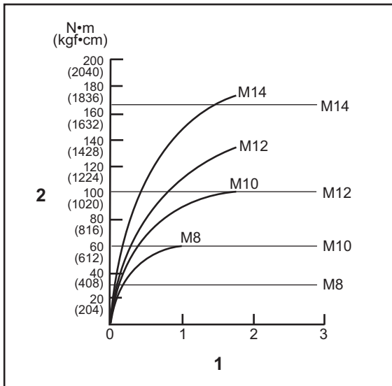
1. Aandraaitijd (seconden) 2. Aandraaimoment
