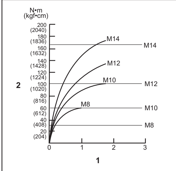
1. Sıkma süresi (saniye) 2. Sıkma torku
